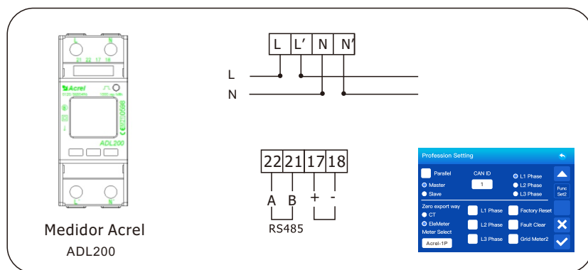
Figura 4.6-1 Conexão do medidor inteligente (fase dividida)
