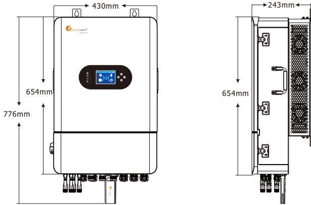
Figura 2.3-2 Dimensões do inversor
