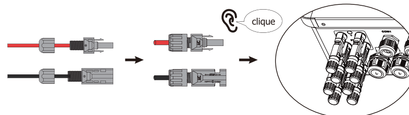
Figura 4.1-4 O plugue FV está conectado ao inversor
