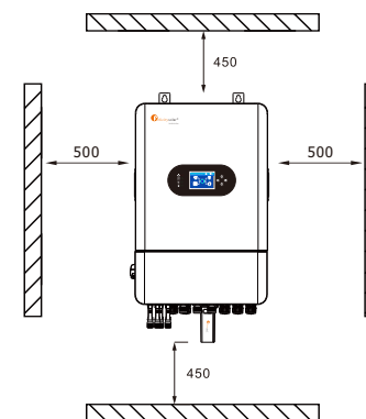
Figura 3.4-1 Espaço de instalação de um inversor
