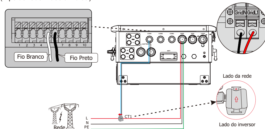
Figura 4.7-1 Conexão CT
