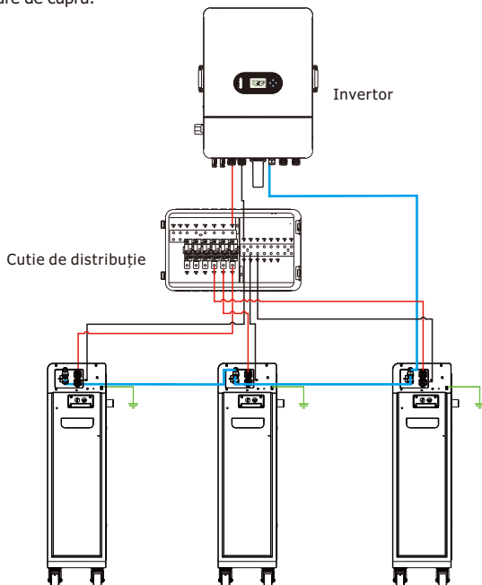
Figura 4-1 Conectarea în paralel a trei acumulatori
