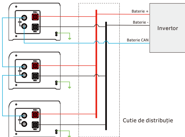
Figura 4-1 Conectarea în paralel a trei acumulatori
