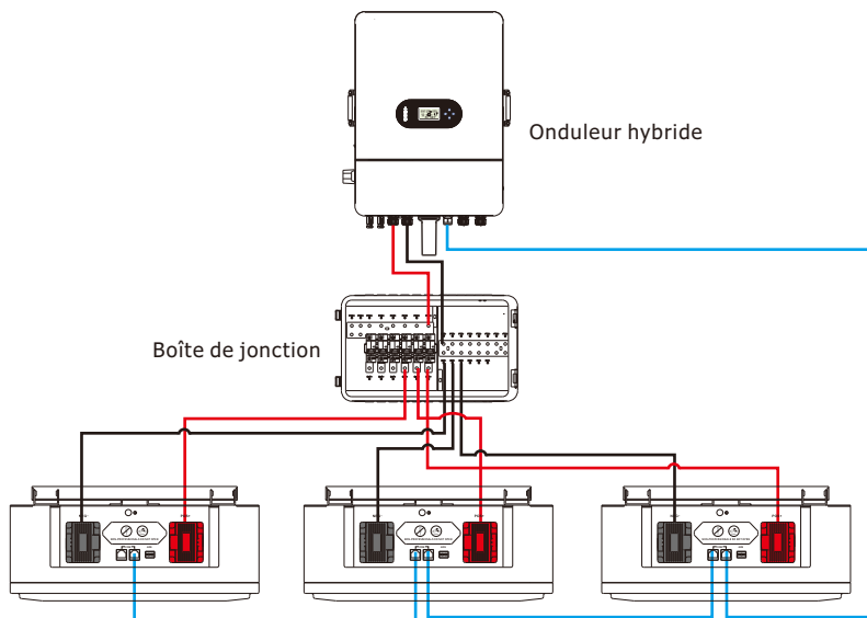
Figure 4-1 : Connexion parallèle de trois blocs batterie
