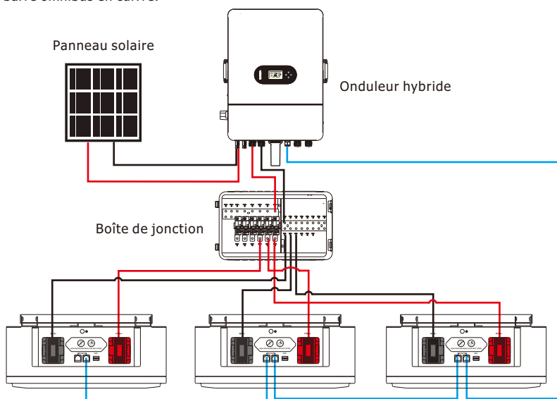
Figure 3-2 : Schéma de connexion d'un système parallèle à plusieurs batteries
