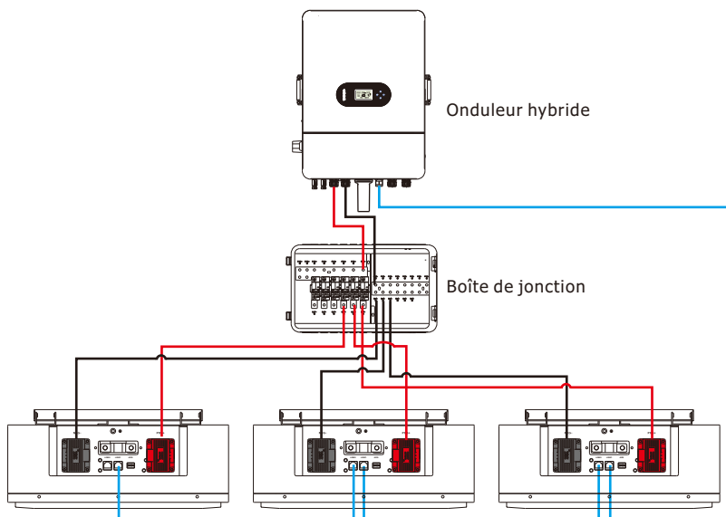
Figure 4-1 : Connexion parallèle de trois blocs batterie
