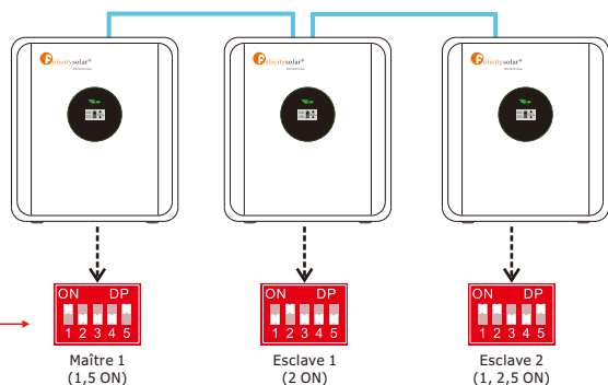
Exemple de trois batteries en parallèle
