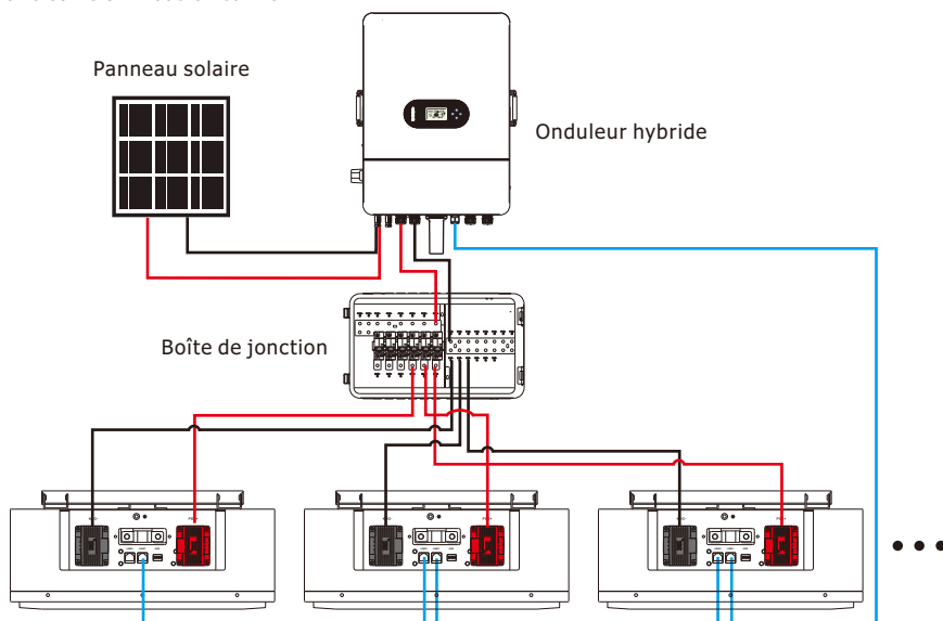
Figure 3-2 : Schéma de connexion d'un système parallèle à plusieurs batteries
