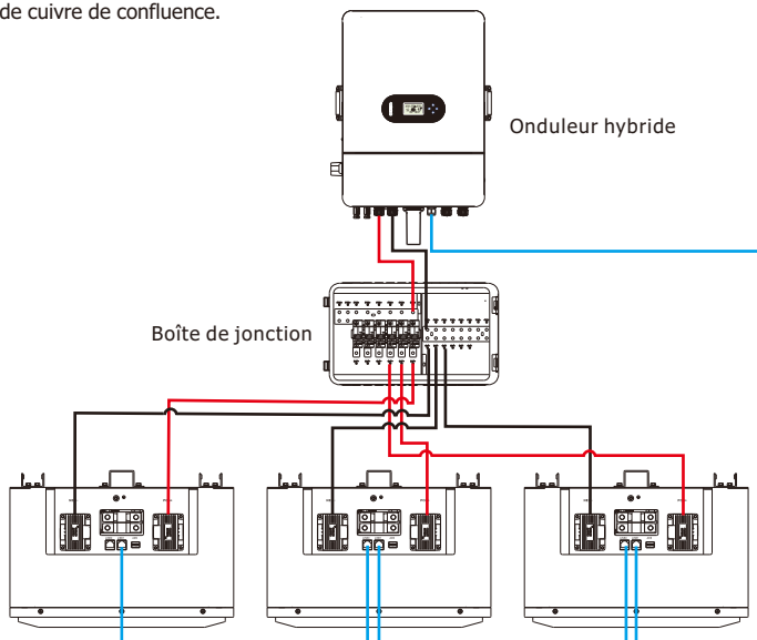
Figure 4-1 : Connexion parallèle de trois blocs batterie
