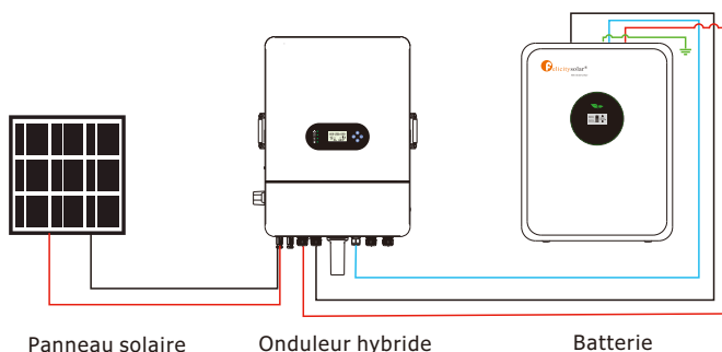
Figure 3-1 : Schéma de connexion d'un système à batterie unique
