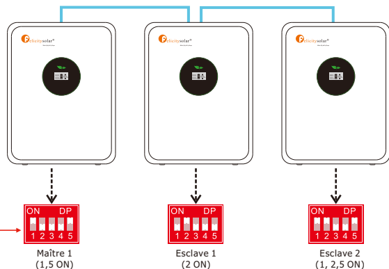
Exemple de trois batteries en parallèle
