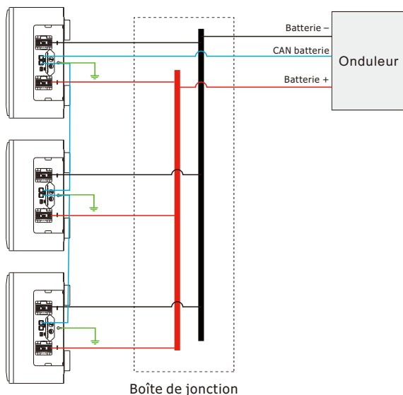
Figure 4-1 : Connexion parallèle de trois blocs batterie
