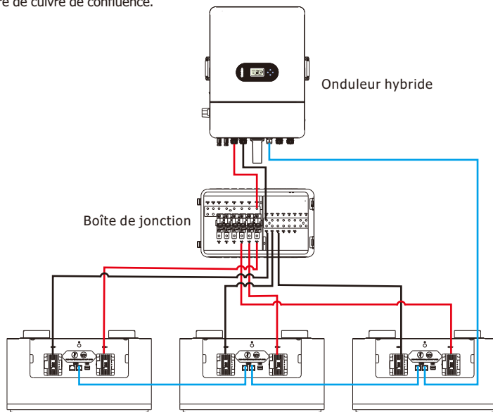
Figure 4-1 : Connexion parallèle de trois blocs batterie
