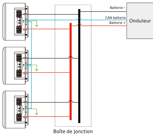
Figure 4-1 : Connexion parallèle de trois blocs batterie
