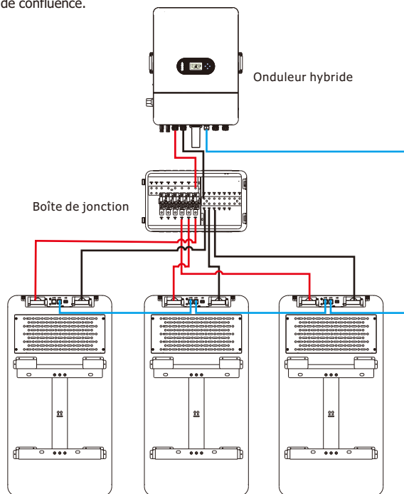
Figure 4-1 : Connexion parallèle de trois blocs batterie
