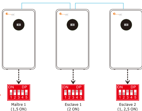
Exemple de trois batteries en parallèle
