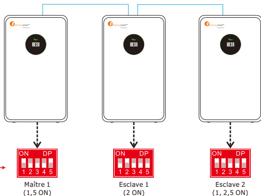
Exemple de trois batteries en parallèle
