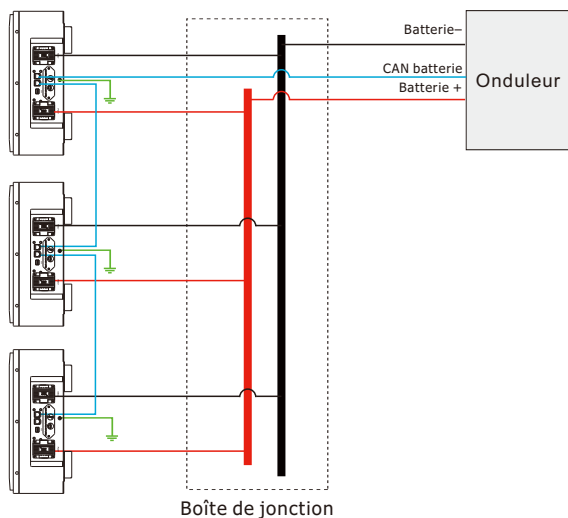
Figure 4-1 : Connexion parallèle de trois blocs batterie
