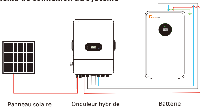
Figure 3-1 : Schéma de connexion d'un système à batterie unique
