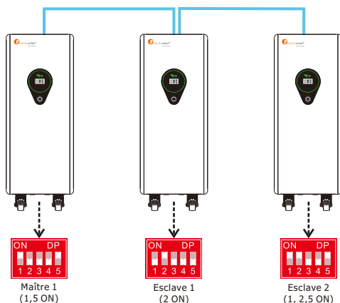
Exemple de trois batteries en parallèle
