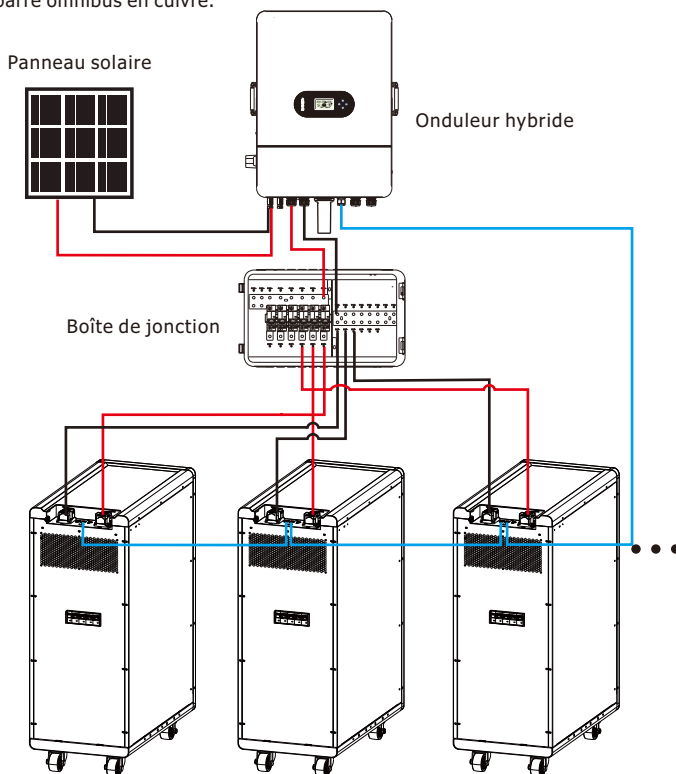
Figure 3-2 : Schéma de connexion d'un système parallèle à plusieurs batteries
