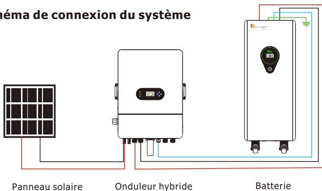
Figure 3-1 : Schéma de connexion d'un système à batterie unique
