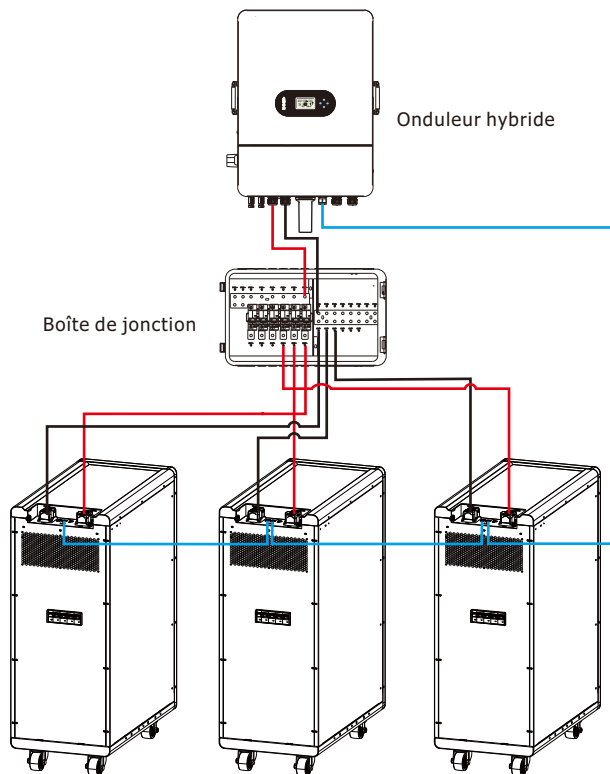
Figure 4-1 : Connexion parallèle de trois blocs batterie
