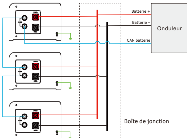
Figure 4-1 : Connexion parallèle de trois blocs batterie
