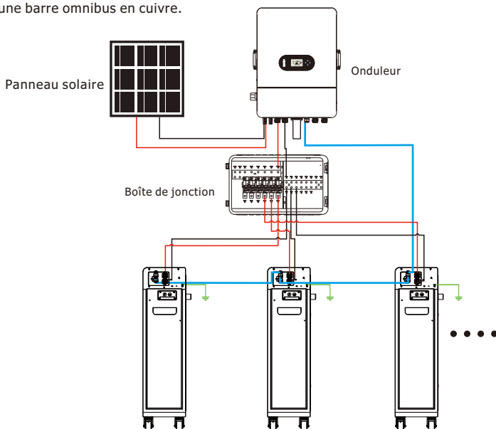
Figure 3-2 : Schéma de connexion d'un système parallèle à plusieurs batteries
