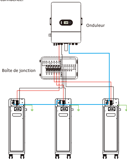
Figure 4-1 : Connexion parallèle de trois blocs batterie
