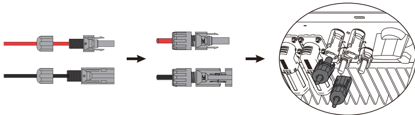
Figure 4.1-3 La fiche PV est connectée à l'onduleur
