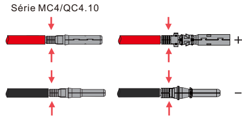
Figure 4.1-2 Câbles PV vers connecteurs PV
