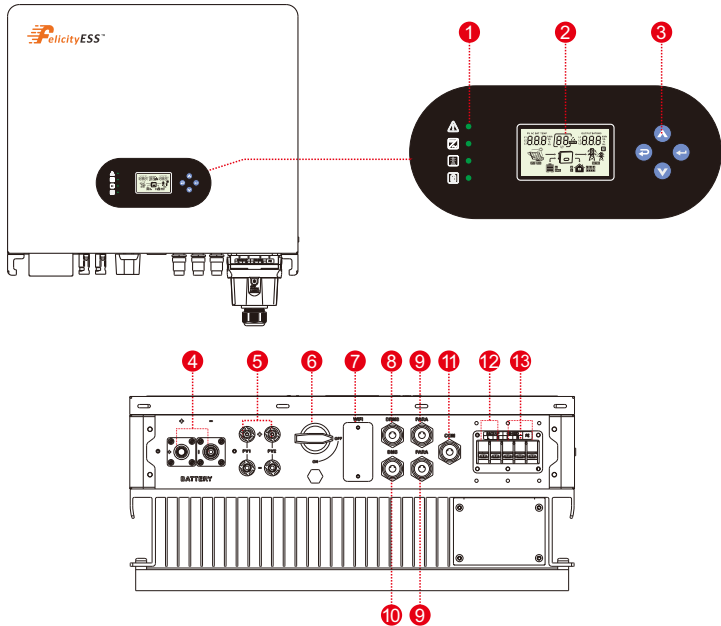
Figure 2.1-1 Présentation des produits
