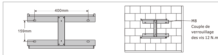
Figure 3.4-1 Installer la plaque de suspension de l'onduleur
