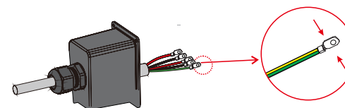
Figure 4.3-5 Installation des bornes de connexion AC
