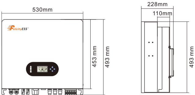
Figure 2.1-2 Dimensions de l'onduleur
