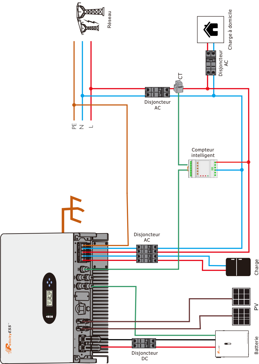
Figure 4.8-1 Système de câblage de l'onduleur
