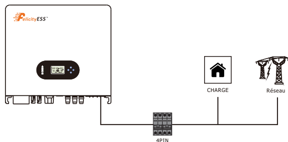
Figure 4.3-2 Connexion du disjoncteur AC
