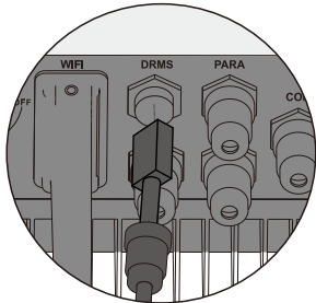
Figure 4.5-2 étapes de fonctionnement
