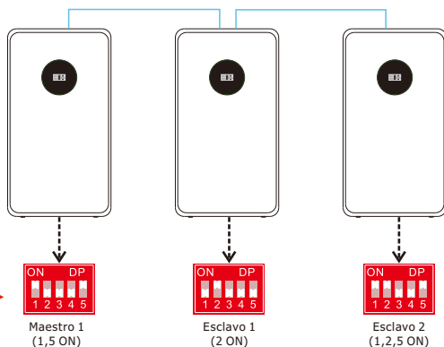
Ejemplo de tres baterías en paralelo
