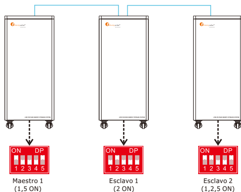
Ejemplo de tres baterías en paralelo
