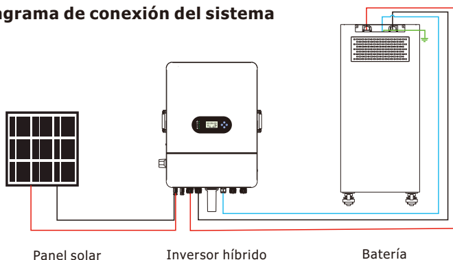
Figura 3-1 Diagrama de conexión del sistema con una sola batería
