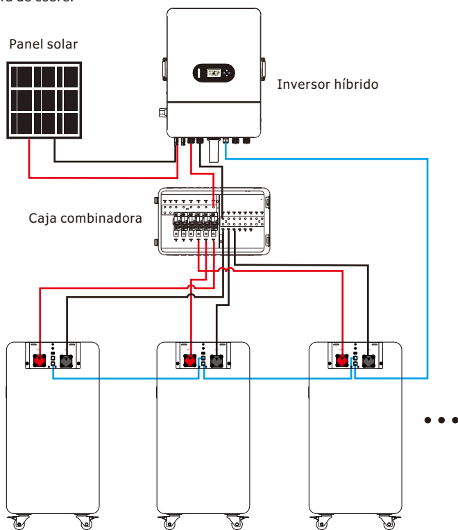
Figura 3-2 Diagrama de conexión de un sistema de baterías múltiples en paralelo
