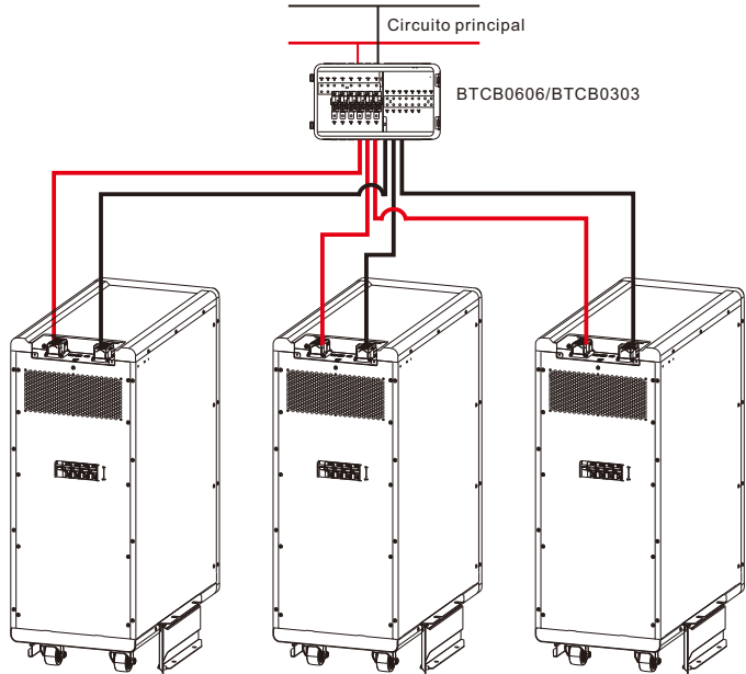
Paso 1: El diagrama esquemático de la conexión en paralelo de tres paquetes de baterías se muestra en la Figura 1.
