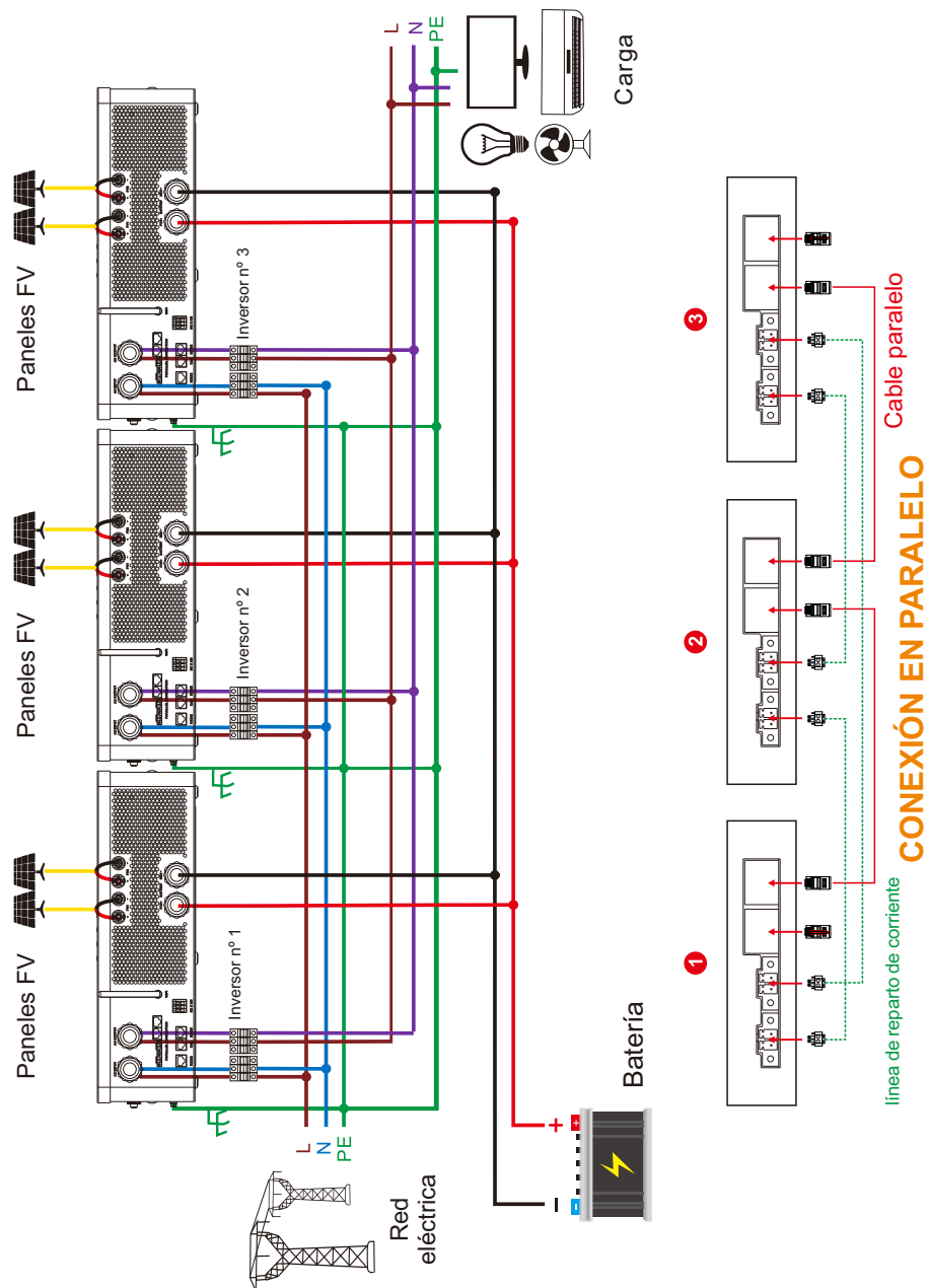
Diagrama de conexión en paralelo monofásica para tres inversores en paralelo
