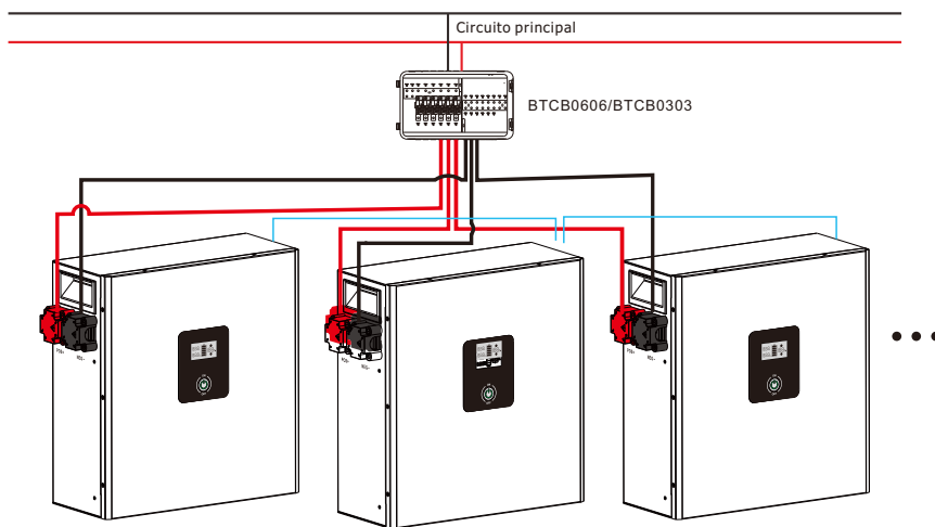
Figura 3-2 Diagrama de conexión de un sistema de baterías múltiples en paralelo
