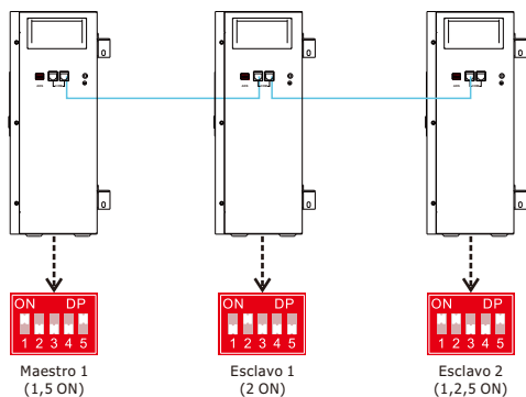
Ejemplo de tres baterías en paralelo
