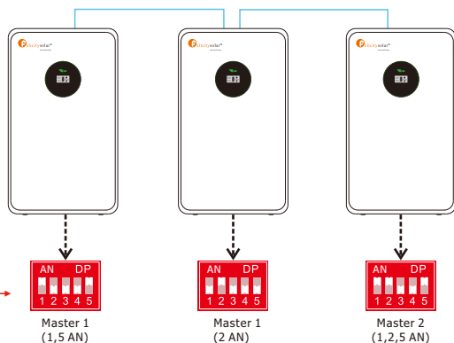
Beispiel für drei parallel geschaltete Batterien
