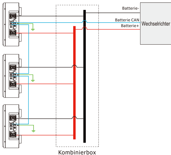
Abb. 4-1 Parallelschaltung von drei Batterien
