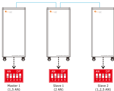
Beispiel für drei parallel geschaltete Batterien
