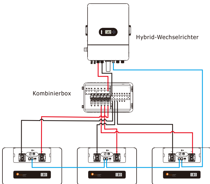
Abb. 4-1 Parallelschaltung von drei Batterien
