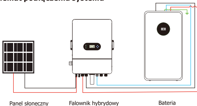
Rysunek 3-1 Schemat podłączenia systemu z jednym akumulatorem
