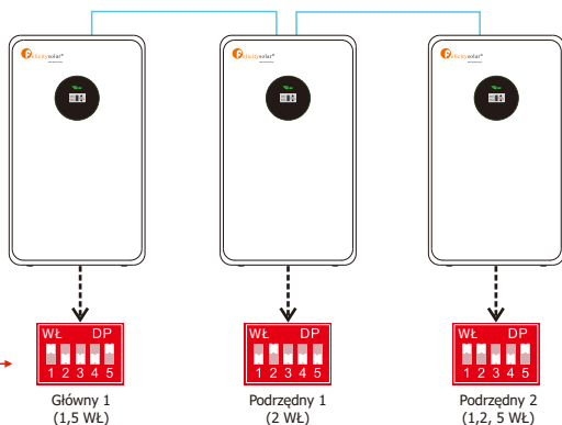
Przykład trzech akumulatorów połączonych równolegle
