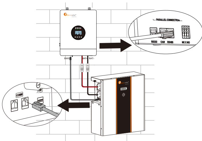
Przypisanie pinów dla portu komunikacyjnego CAN/RS485 inwertera
