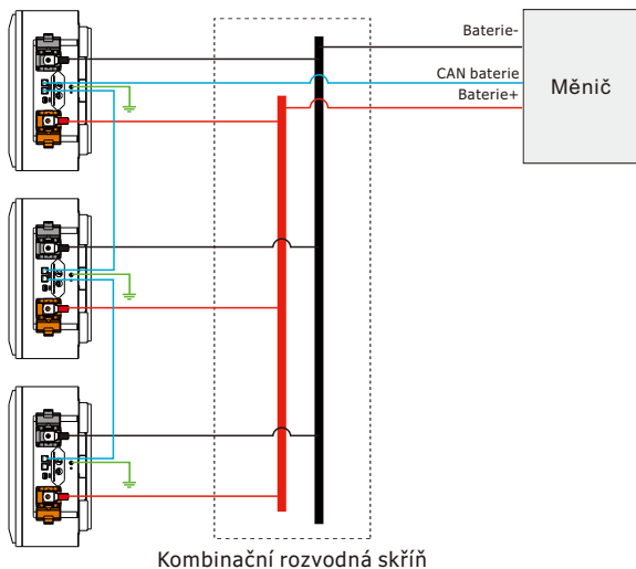
Obrázek 4-1 Paralelní zapojení tří bateriových modulů
