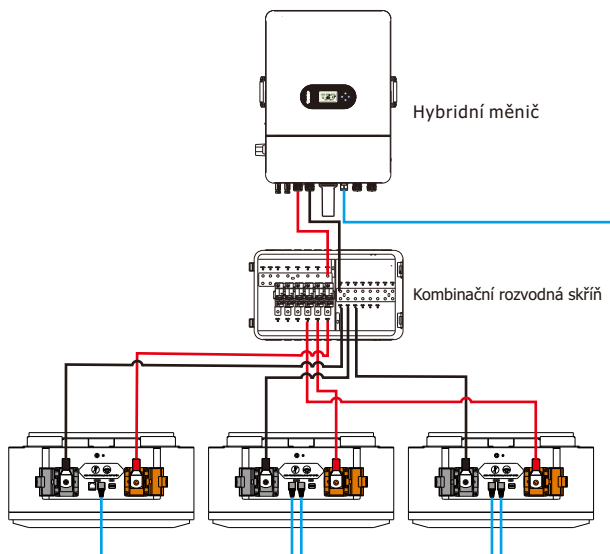
Obrázek 4-1 Paralelní zapojení tří bateriových modulů
