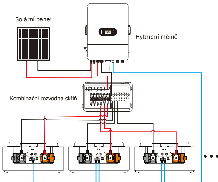
Obrázek 3-2 Schéma zapojení paralelního systému více baterií
