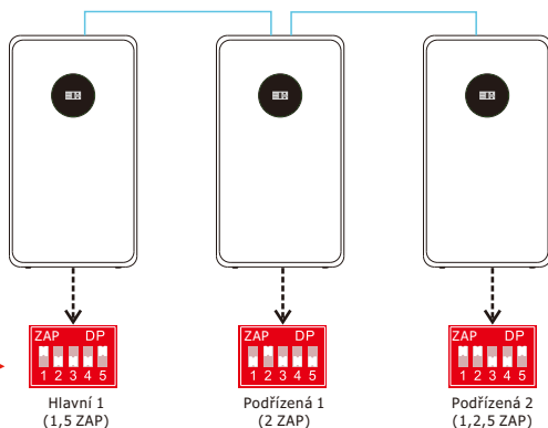
Příklad tří baterií zapojených paralelně
