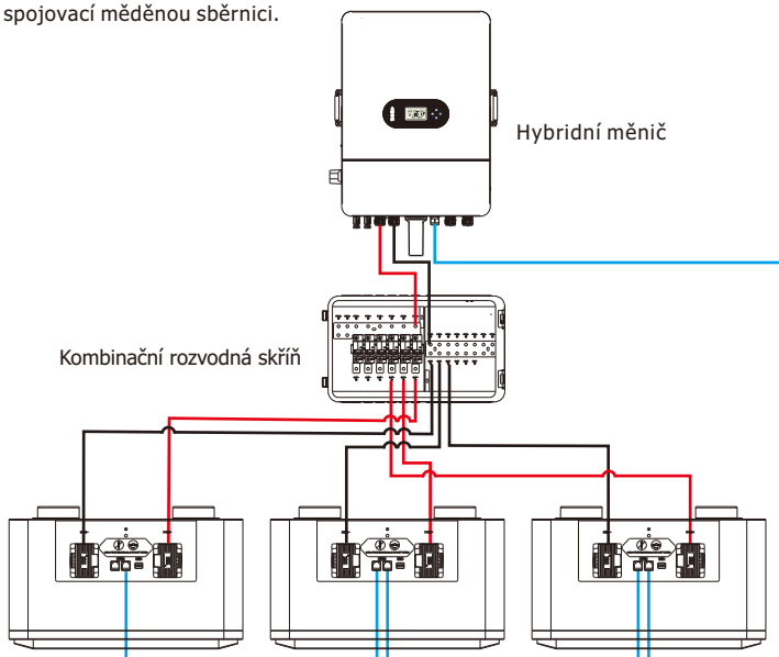
Obrázek 4-1 Paralelní zapojení tří bateriových modulů
