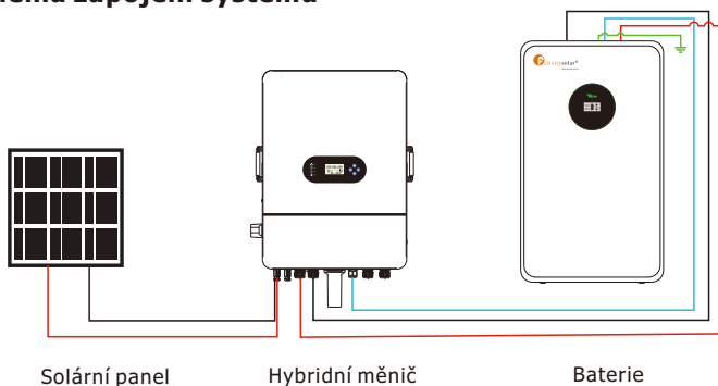
Obrázek 3-1 Schéma zapojení jediné bateriové soustavy
