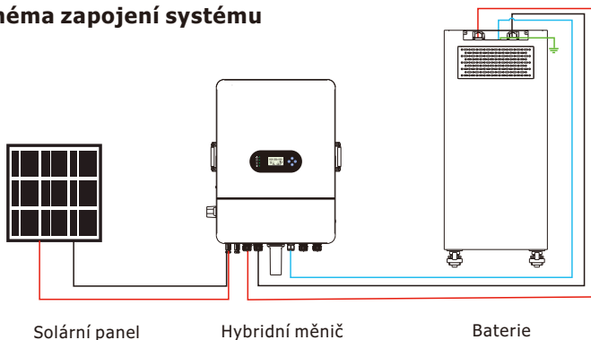
Obrázek 3-1 Schéma zapojení jediné bateriové soustavy
