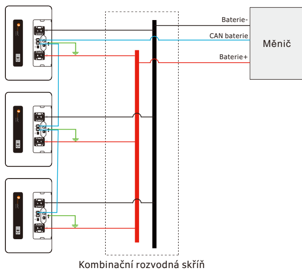
Obrázek 4-1 Paralelní zapojení tří bateriových modulů
