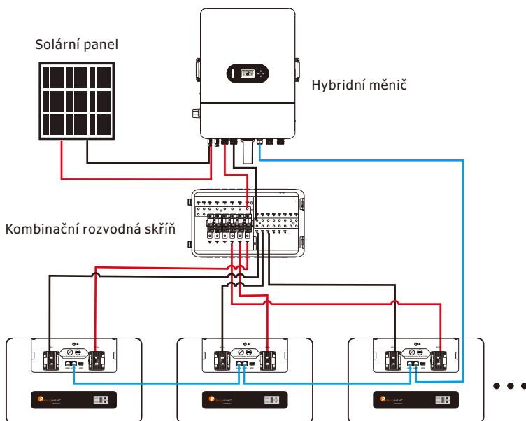
Obrázek 3-2 Schéma zapojení paralelního systému více baterií
