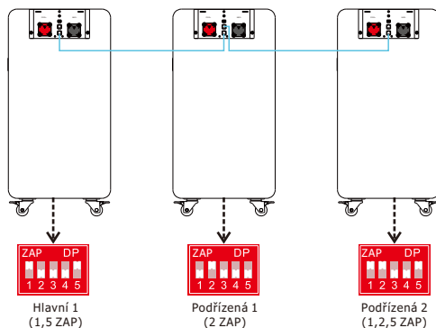
Příklad tří baterií zapojených paralelně
