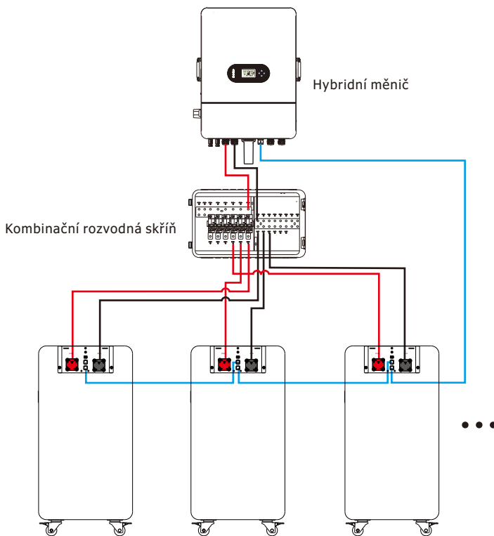
Obrázek 4-1 Paralelní zapojení tří bateriových modulů
