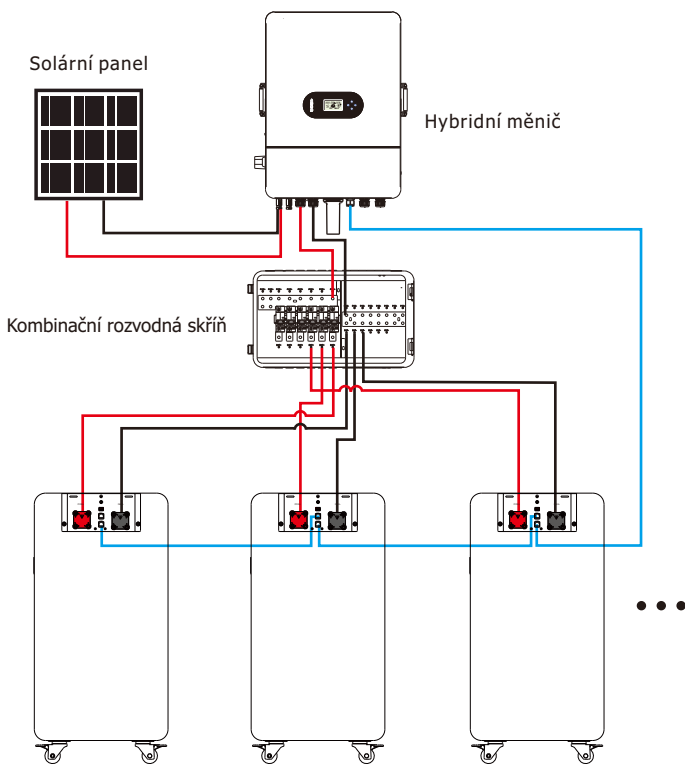
Obrázek 3-2 Schéma zapojení paralelního systému více baterií
