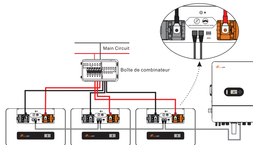
Figure 1 : La connexion en parallèle de trois packs de batteries
